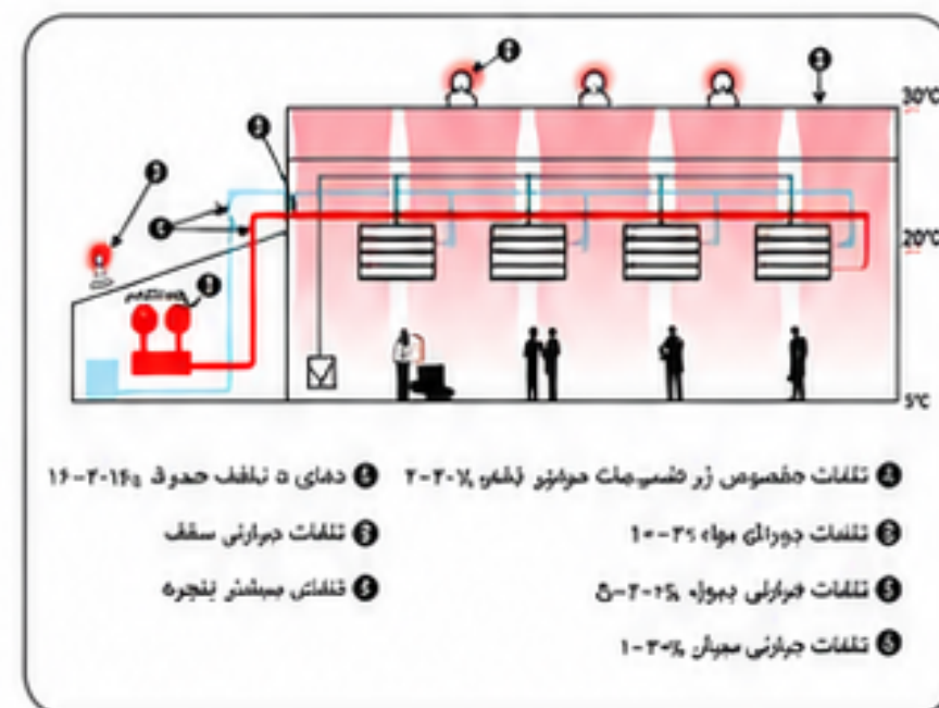
معایب سیستم های گرمایش همرفتی
