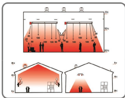
امکان منطقه بندی دمایی و تمرکز گرما بر کف سالن در سیستم گرمایش تابشی
