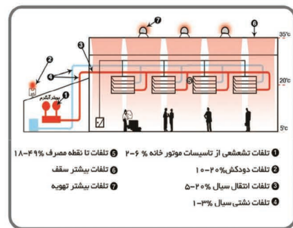
معایب سیستم های گرمایش همرفتی
